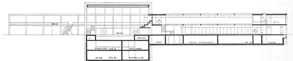
Schnitt C
