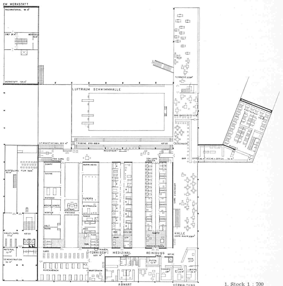
1. Stock 1 : 700
