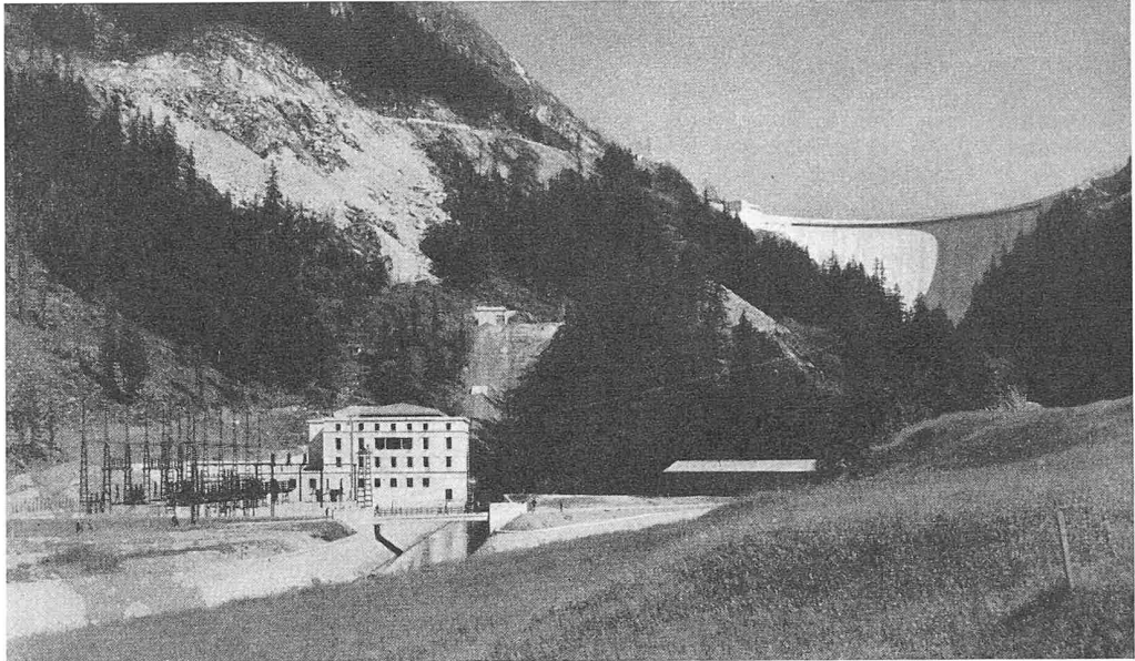
Bild 35 (rechts). Zentrale Les Brévières mit Staumauer Tignes
