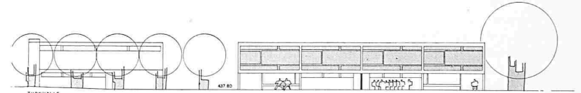
Südansicht, Erdgeschoss und Obergeschoss, 1 : 700
