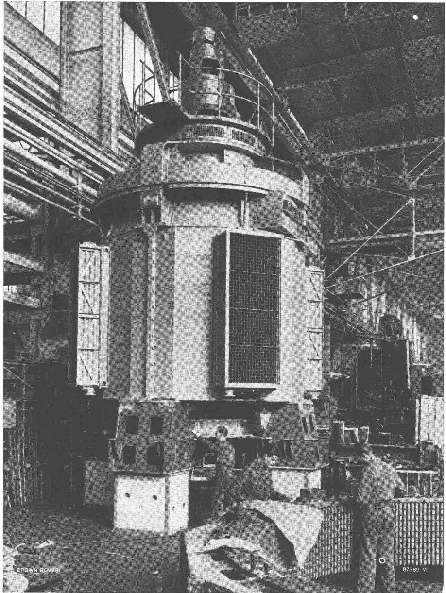
Einer der drei vertikalachsigen 60 000-kVA-Generatoren für die Zentrale Fionnay der Kraftwerke Mauvoisin AG., Sitten, Wallis, bei seiner Fertigstellung in der grossen Montagehalle.
