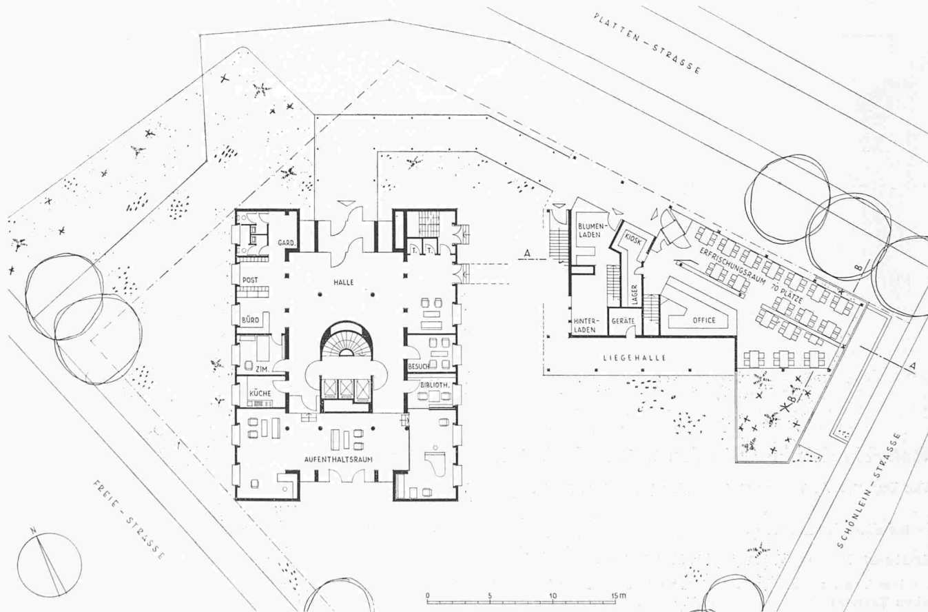
Erdgeschoss von Hochhaus und Anbau
