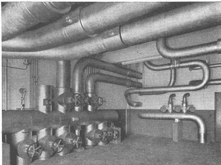
Technische Anstriche in der chemischen Industrie. Apparate und Röhren mit Aluminiumbronze 400° hitzebeständig gestrichen. Wandanstriche mit ECLASIT sind resistent gegen chem. Dämpfe.
