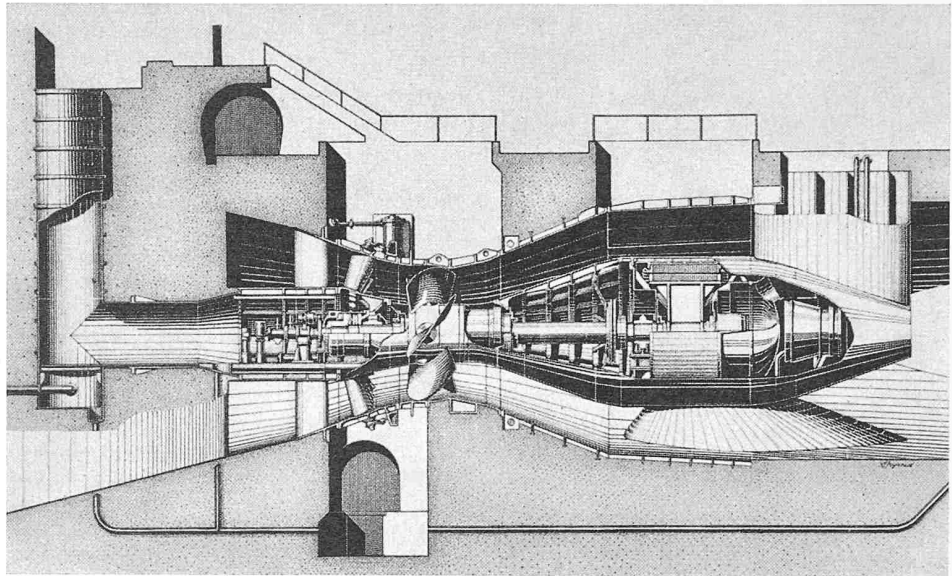
Bild 105. Kraftwerk Argentat, Schnitt durch eine Rohrturbinen-Gruppe
