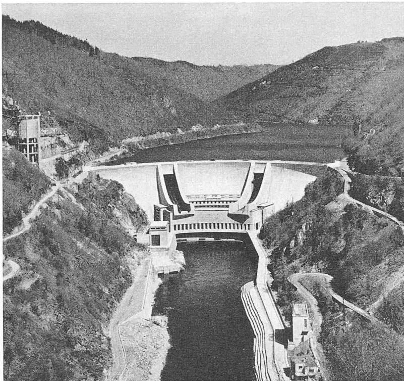
Bild 98. Hochwasser-Entlastung im Betrieb
