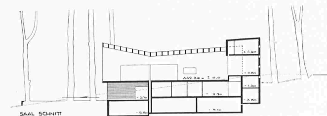
SAAL SCHNITT
