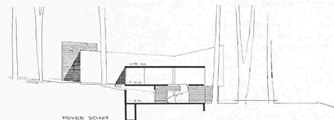
FOYER SCHNITT
