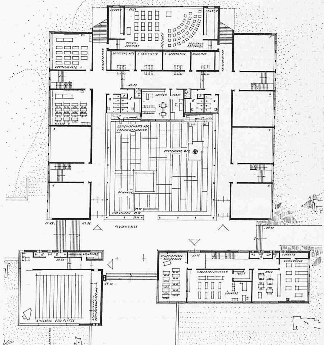
Schulhaus, Erdgeschoss
