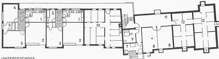
Block 2, Grundrisse und Schnitte 1:400. 1 Küche, 2 Wohnzimmer, 3 Schlafzimmer, 4 Zimmer, 5 Bad, 6 WC, 7 Waschküche, 8 Trockenraum, 9 Heizung, 10 Abstellräume, 11 Einstellraum, 12 Keller- und Luftschutzraum
