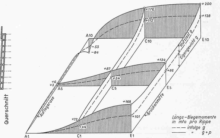
Bild 8. Momentenfläche für Eigengewicht und Nutzlast
