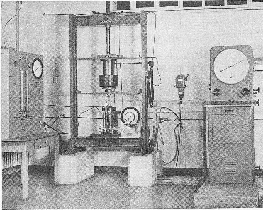
Bild 6 (rechts). Grosser triaxialer Scherapparat zur Untersuchung der Stützkörpermaterialien für Probengrößen von 90 cm Höhe und 2000 cm 2 Querschnittsfläche
