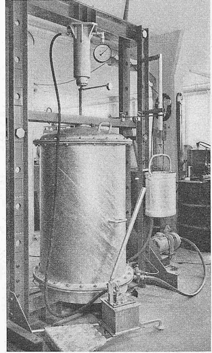
Bild 6 (rechts). Grosser triaxialer Scherapparat zur Untersuchung der Stützkörpermaterialien für Probengrößen von 90 cm Höhe und 2000 cm 2 Querschnittsfläche
