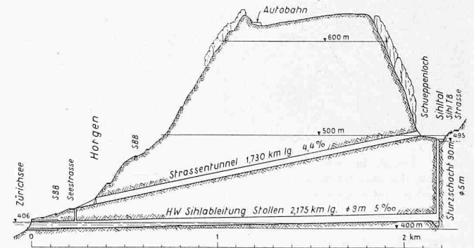
Bild 2. Längenprofil (fünffach überhöht) der Hochwasserableitung der Sihl in den Zürichsee. Oberhalb des Sihlstillens kann ein Strassentunnel angelegt werden, welcher als Basisverbindung von den Seestrassen (Fähre Horgen - Meilen) zur Sihlthalstrasse und Autobahn Zürich - Süd und zur Innerschweiz dienen könnte.
