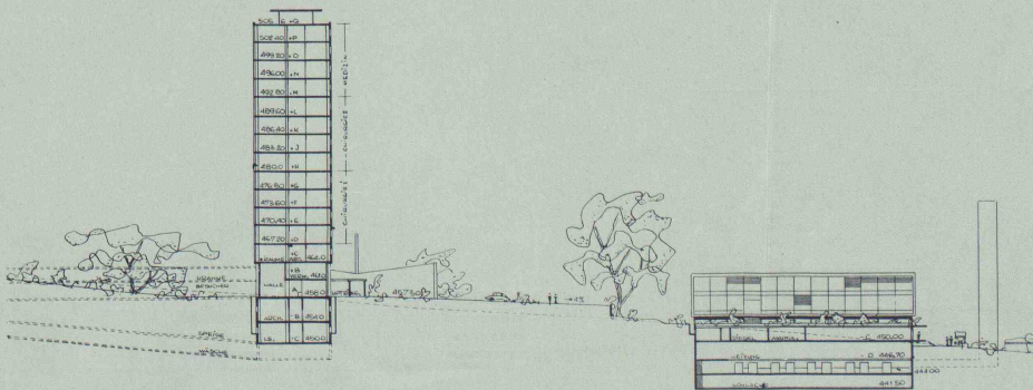
Querschnitt Bettenhaus, M. 1:1000
