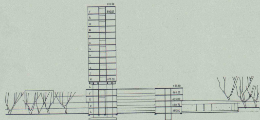
Stadspital Querschnitt, M. 1:1000
