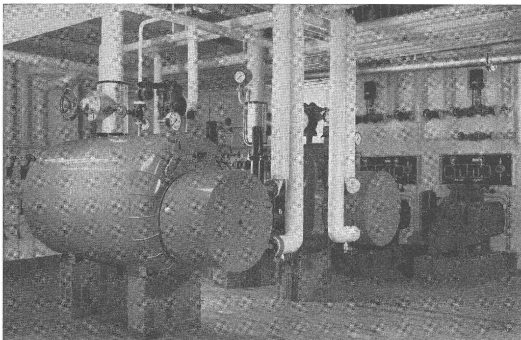
Heißwasser-Dampfumformer
