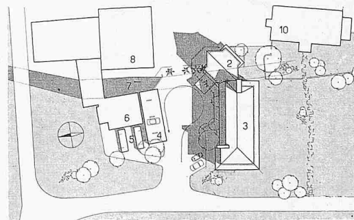
Lageplan M 1 : 2000 1 Eingang, 2 Ausstellungshalle, 3 Bürotrakt, 4 Autounterstand, 5 Velounterstände, 6 Lager, 7 Rautibach, 8 Fabrikkantäne, 9 Werkstatt, 10 Alter Verwaltungsbau
