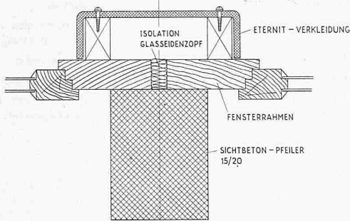
Pfeilverkleidungen, Horizontalschnitte 1:8
