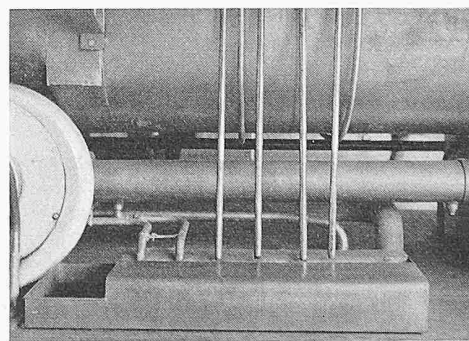
Bild 14. Gefäss aus verzinnem Kupferblech zum Auffangen von Kondenswasser und Abdampf der Mangel mit sichtbarem Abfluss
