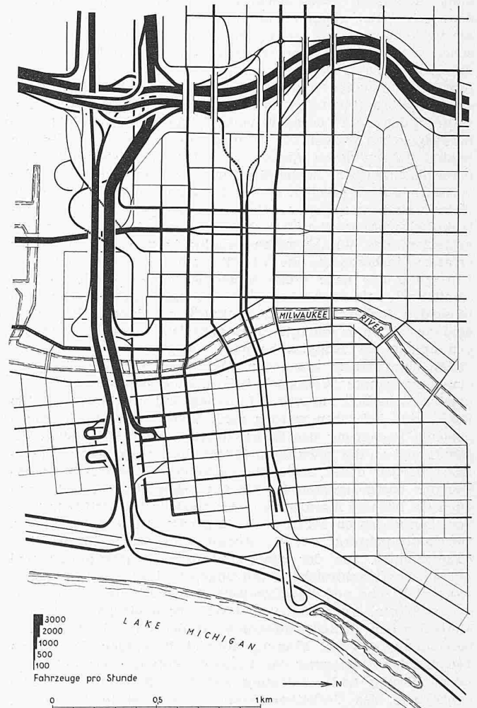
Bild 5. Das gleiche Gebiet, Spitzenbelastung 1980, falls die Expressstrassen gebaut werden. — Untersuchungen des Büros Ammann & Whitney, New York
