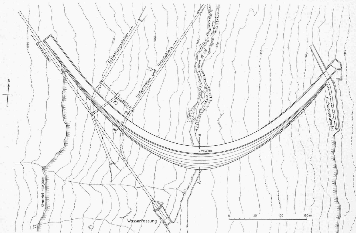
Bild 4. Die Staumauer Lei, Grundriss 1:4000
