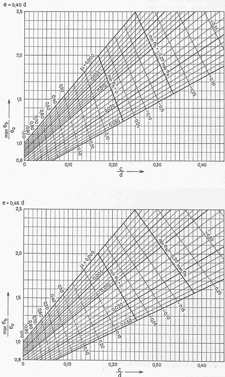
Bild 3. Symmetrisch armierter Rechteckquerschnitt unter Längskraft mit Biegung (kleine Exzentrizität) im elastischen Bereich; n = 10
