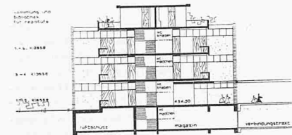
Schnitt Schulhaus 1:700
