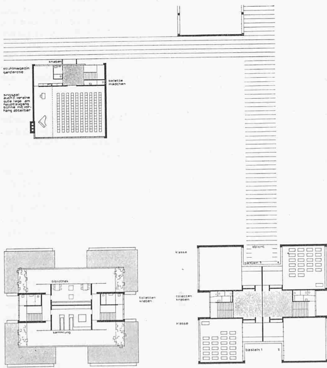
Obergeschoss
