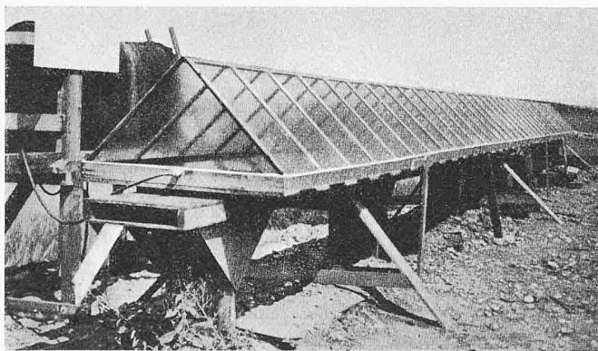
Bild 14. Sonnen-Destillier-Anlage
