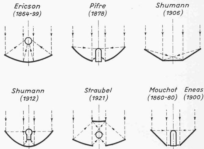
Bild 12. Ausgeführte Spiegelformen
