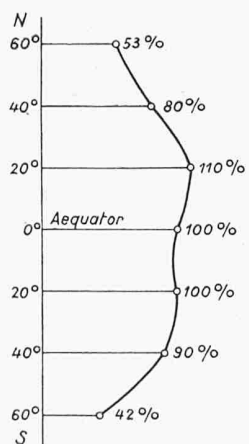
Bild 1. Verteilung der mittleren Sonneneinstrahlung über die geographische Breite. Einstrahlung am Aequator = 100 %
