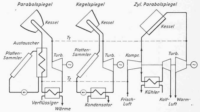
Bild 20. Drei Beispiele typischer Schaltungen von Sonnenkraftanlagen
