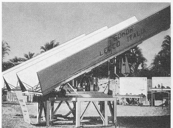
Bild 21. Italienische Sonnenkraftmaschine
