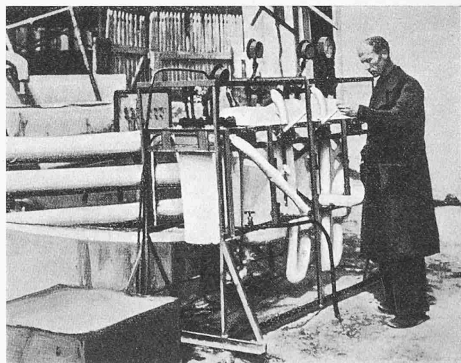
Bild 15 (rechts). Russische Ausführung einer mehrstufigen Destillierbatterie zur Süßwassergewinnung
