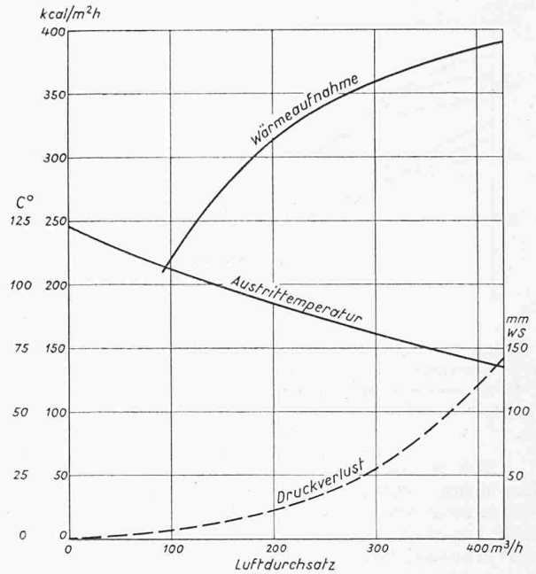
Bild 8. Plattensammler für Lufterwärmung. Luftaustrittstemperatur, Druckverlust und Wärmeaufnahme in Abhängigkeit des Luftdurchsatzes
