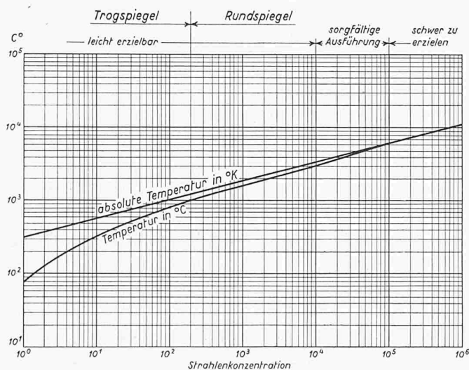
Bild 11. In der Brennpunktzone eines Strahlenkonzentratoren erzielbare Temperaturen in Abhängigkeit der Strahlenkonzentration
