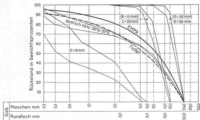
Bild 1. Streuungsbereiche der drei lieferbaren Komponenten eines gut eingerichteten zürcherischen Kieswerkes. Gefährlich ist die grosse Schwankung der Komponenten 0 ÷ 8 mm. Gewichtsmässige Dosierung der Zuschlagstoffe ist für Qualitätsbeton, und sei es mengenmässig noch so wenig, notwendig
