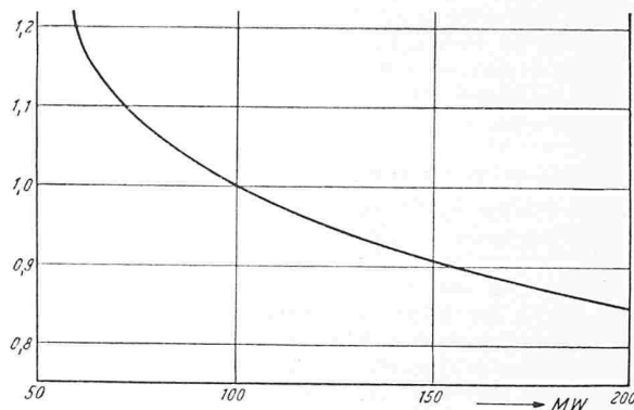
Bild 7. Abnahme der verhältnismässigen Baukosten von CH-Reaktoren mit zunehmender elektrischer Leistung des Kraftwerks pro Kernreaktor.
