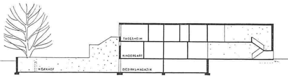
Längsschnitt Tagesheim
