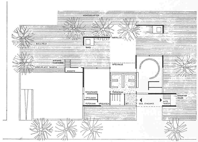
ERDGESCHOSS KINDERGARTEN Erdgeschoss Kindergarten 1:700
