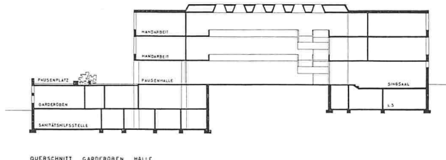
Schnitt Nord-Süd durch Halle
