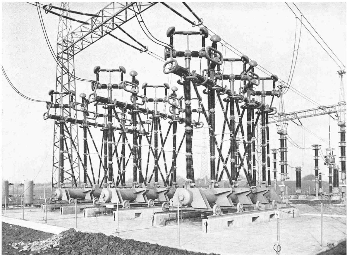
Bild 4. 400 kV Druckluftschnellschalter in der Anlage Hoheneck des Rheinisch-Westfälischen Elektrizitätswerkes (RWE). Diese Schalterausführung bewältigt eine Ausschaltleistung von 20 000 MVA symmetrisch einwandfrei
