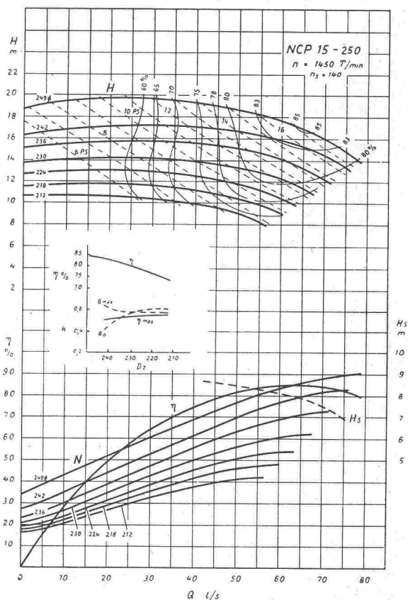
Kennlinien einer Spiralgehäusepumpe mit verschiedenen Laufraddurchmessern
