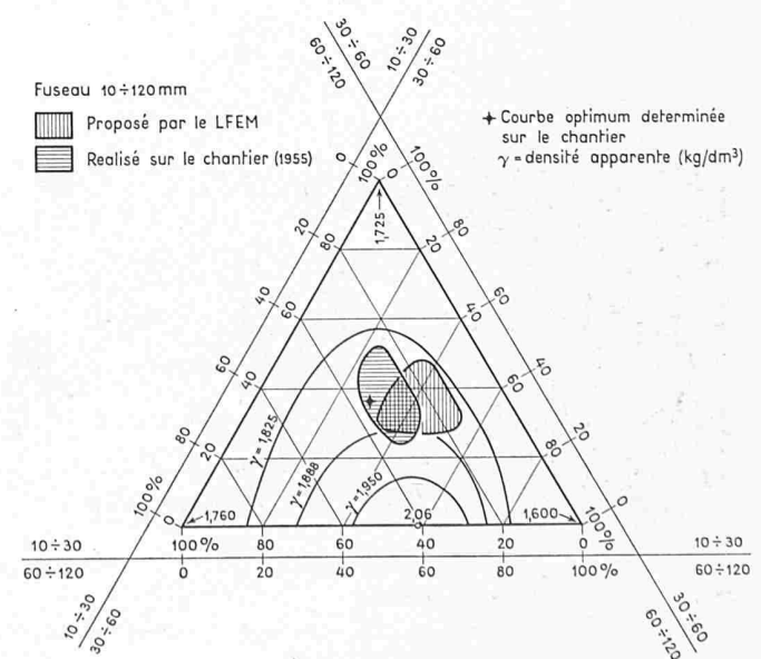
Fig. 17. Densité apparente de différents mélanges de 10 ÷ 30, 30 ÷ 60 et 60 ÷ 120 mm
