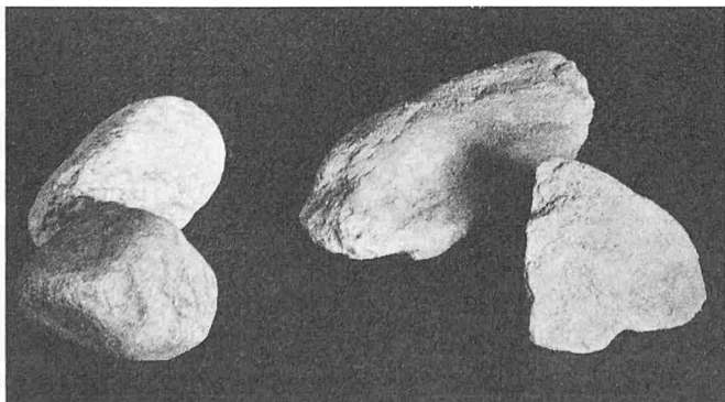
Fig. 8. Empoussièremment des agrégats entre la sortie du lavage-triage (à gauche) et le silo de la tour à béton (à droite)
