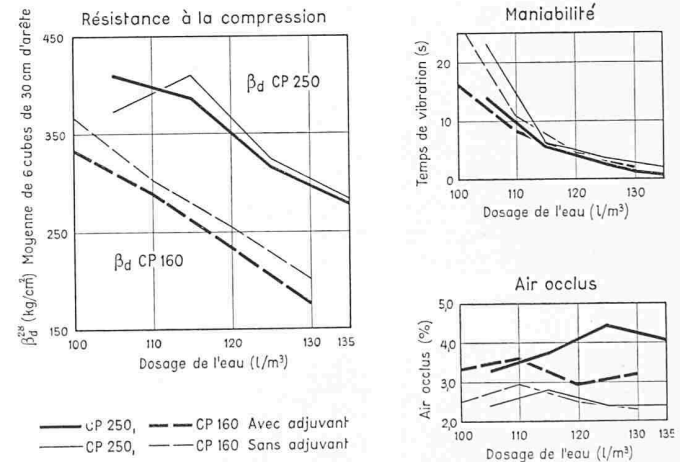
Fig. 2. Dosage de l'eau
