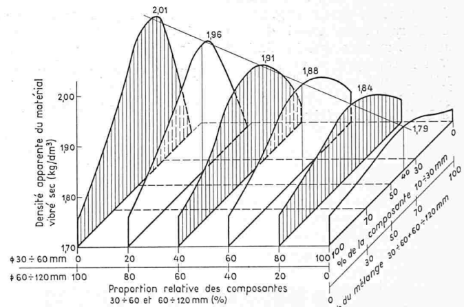
Fig. 16. Densité apparente de différents mélanges de 10 ÷ 30, 30 ÷ 60 et 60 ÷ 120 mm
