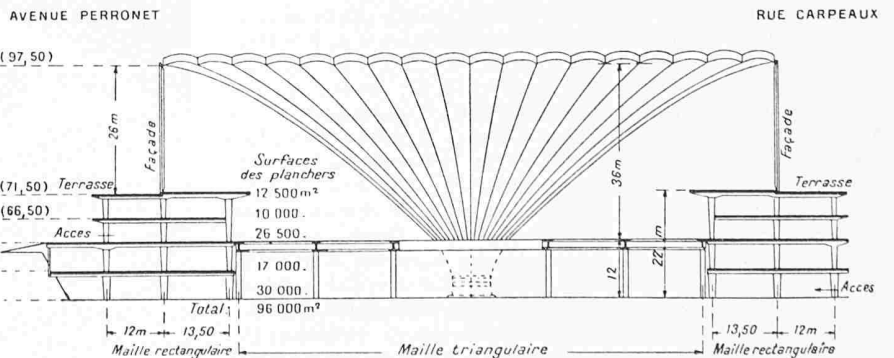
Schnitt 1:1500 durch die Böden im Dreiecknetz (Mitte) und in den Seitenbauten mit Rechteckgrundriss (ausen)
