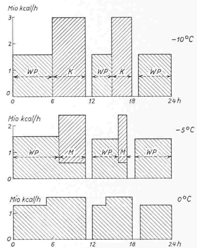
Bild 4. Heizprogramme für mittl. Tages-temperaturen von -10 , -5 und 0^{\circ}\text{C} . WP = Wärmepumpenbetrieb, K = Kesselbetrieb, M = gemischter Betrieb
