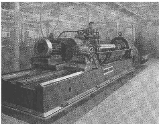
Walzenschleifmaschine auf isoliertem Fundament
