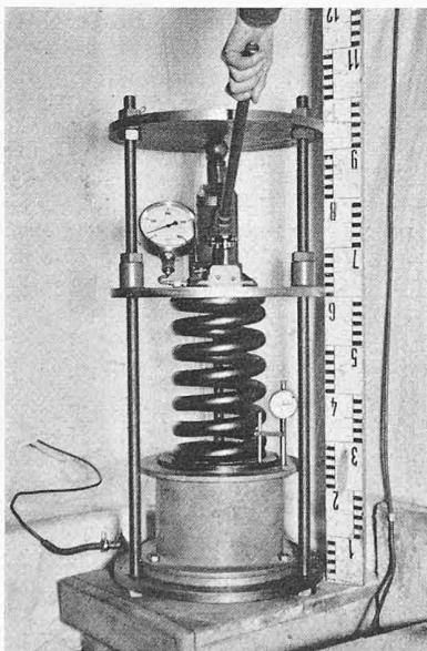
Bild 4. Oedometer für Proben mit 500 cm 2 Grundfläche und 20 cm Höhe. Der Proctorzylinder dient zugleich dem Proctor-Verdichtungsversuch.
