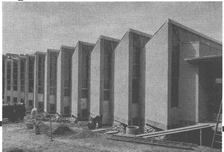
Eisenbetonbau, vollständig mit PORA-Platten ummantelt
