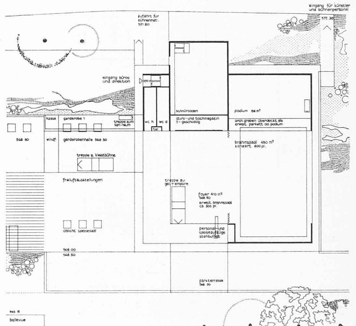
Erdgeschoss 1:800
