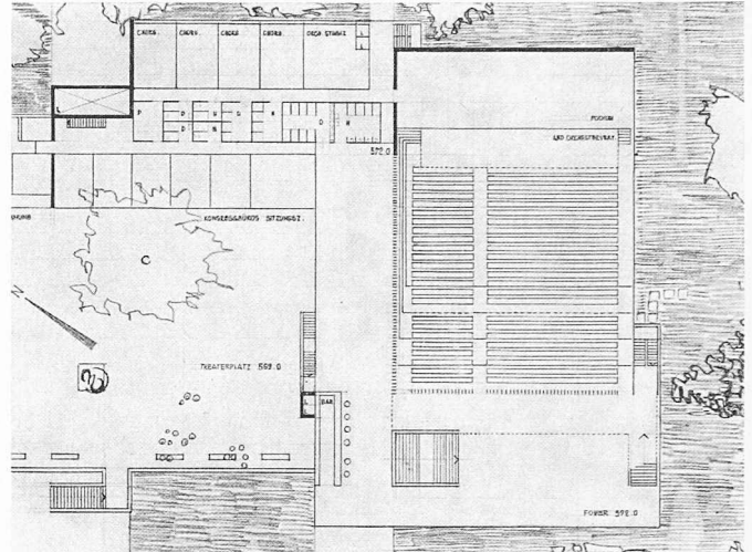
Erdgeschoss 1:800, Brahmssaal
