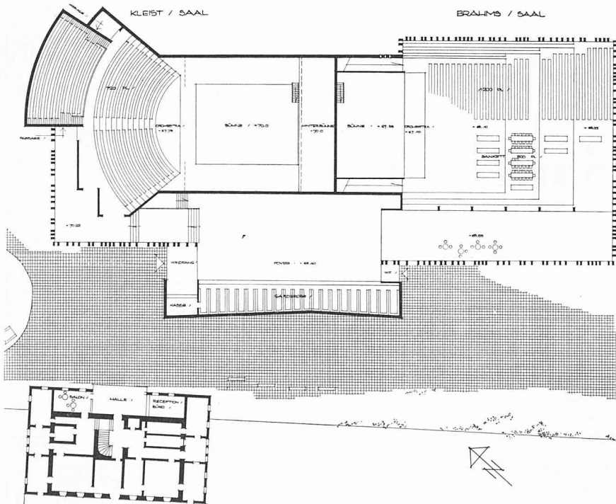
Erdgeschoss 1:800
