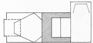
EG. NUR THEATER
