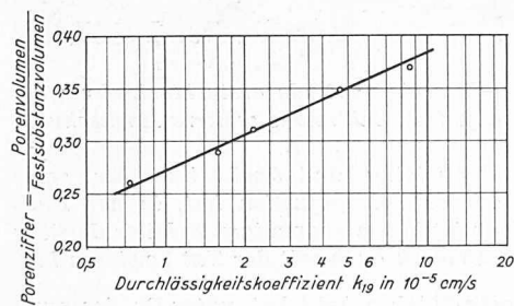
Links: Zusammenhang zwischen der Durchlässigkeit und der Porenziffer des Kernmaterials
