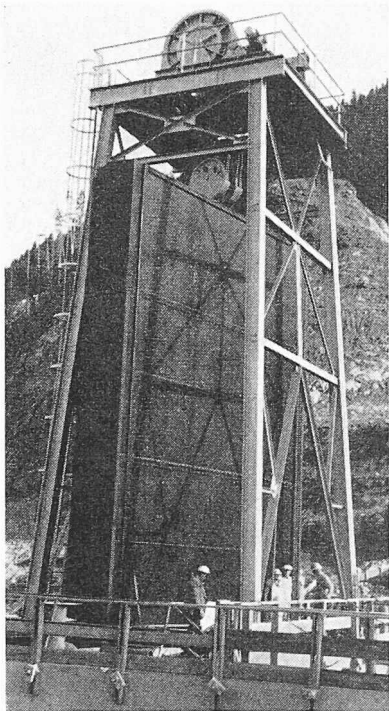
Bild 19. Swift-Damm, aufgezogene Hubschütze der Wasserfassung
