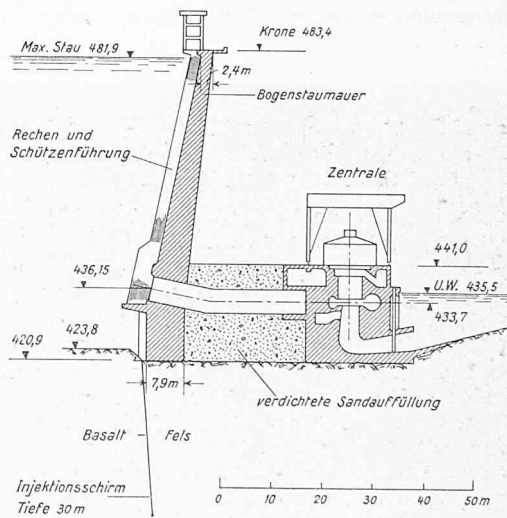
Bild 28. Pelton, Querschnitt 1:1500 durch Staumauer und Zentrale
