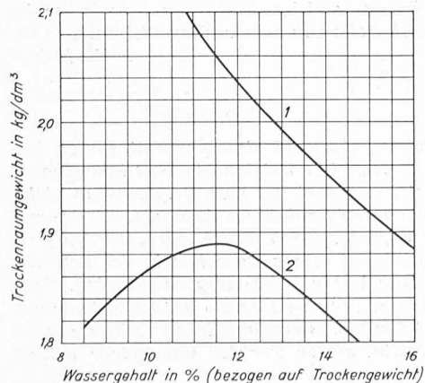
Bild 16. Swift-Damm, Materialkonstanten
