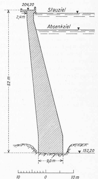
Schnitt A-A
