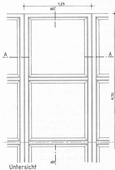
Bild 3. Rippenplatten, Deckenelemente 1:40
