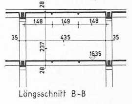
Bild 12 (links). Industriebau für Elektromotoren, Grundriss und Schnitt 1:200. Nutzlast 750 bis 1000 kg/m 2
