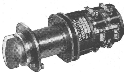
Kommandoschalter Typ N1 10 für 10 A 500 V
