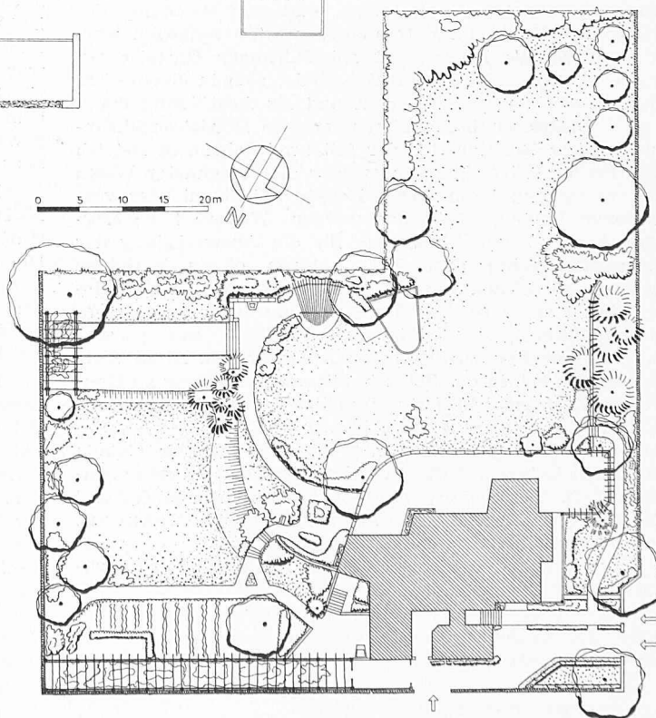
Lageplan 1:800
