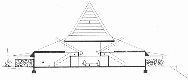
Querschnitt
