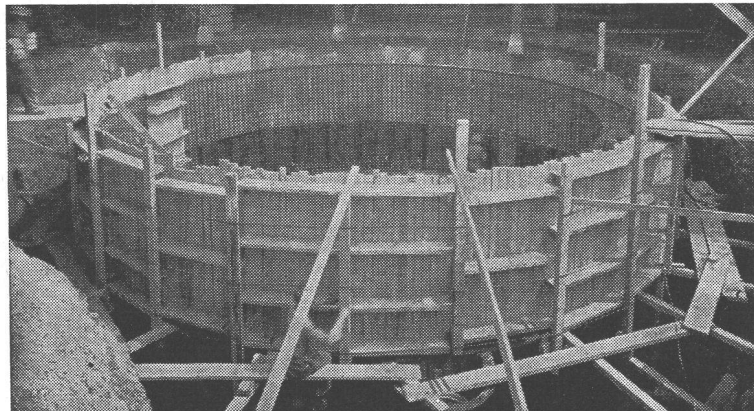
Betonfank von 250 000 l im Bau
