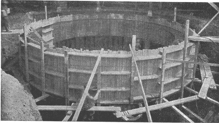
Betonfank von 250 000 l im Bau
