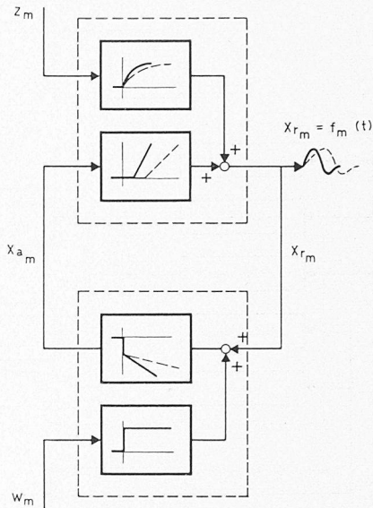
b) Analogiesystem
