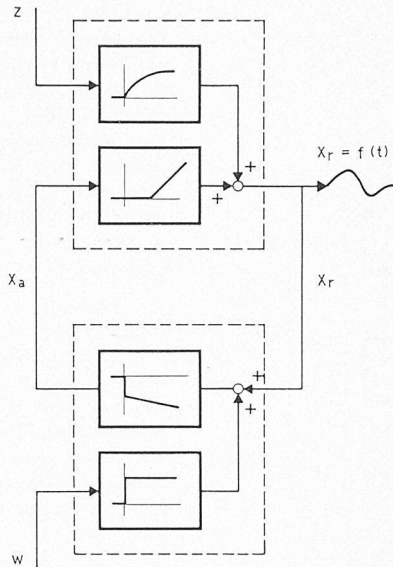
a) Originalsystem
