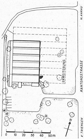
Bild 1. Lageplan 1:2500
