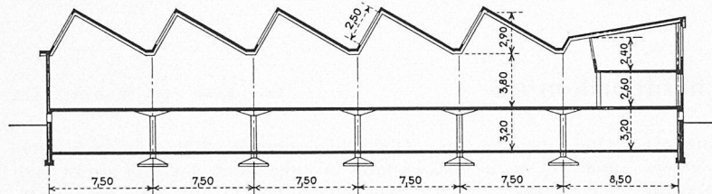
Bild 4. Längsschnitt 1:500
