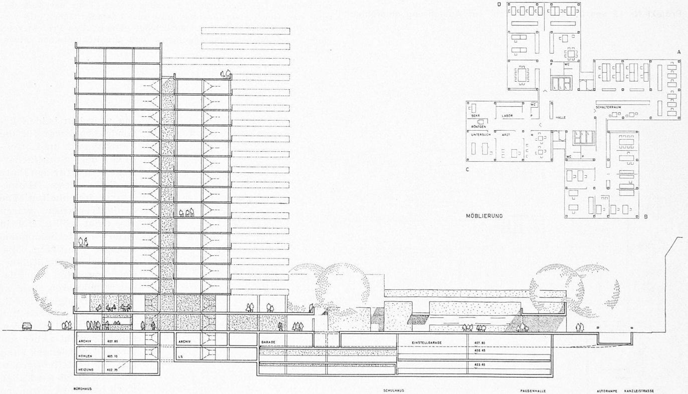
Schnitt Nordost-Südwest, 1:700
