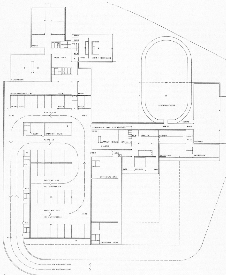
Untergeschossgrundriss 1:700
