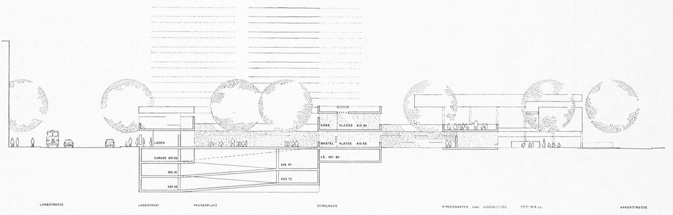
Schnitt Nordwest-Südost
