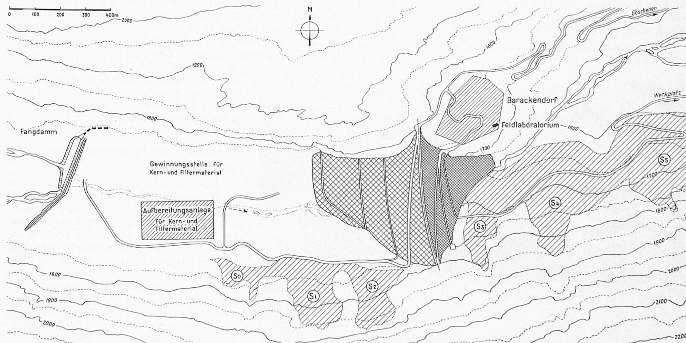
Bild 2. Uebersicht, 1:15 000, über die Baustelle: Staudamm, Barackendorf (Feldlabor), Gewinnungsstellen für Kern- und Filtermaterialien (Talboden) sowie für Stützkörpermaterialien (Schutthalden S 0 bis S 5 ), Aufbereitungsanlage
