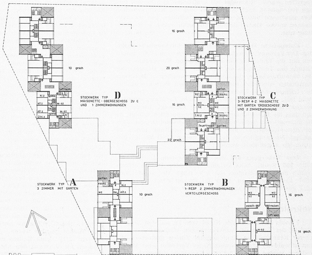
Wohnungsgrundrisse 1:1000
