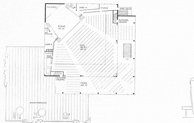
Saalgeschoss 1:700
