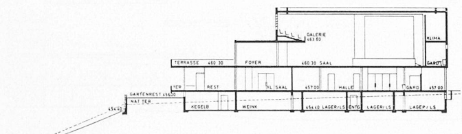
Schnitt B-B
