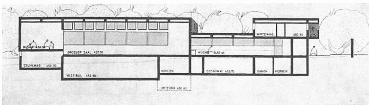
Schnitt Nord-Süd
