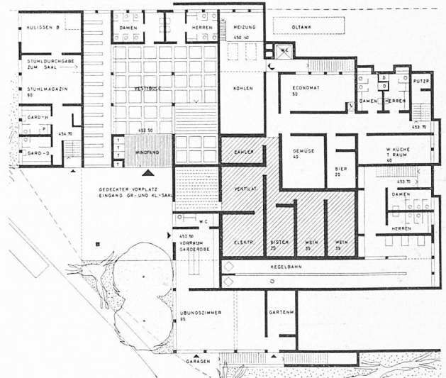
Untergeschoss 1:700
