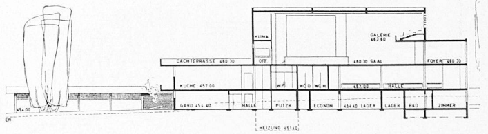
Schnitt A-A
