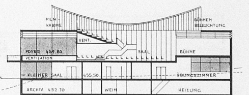
SCHNITT B - B
