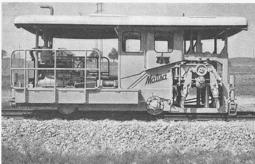
Bild 12. Selbstfahrende Krammmaschine
