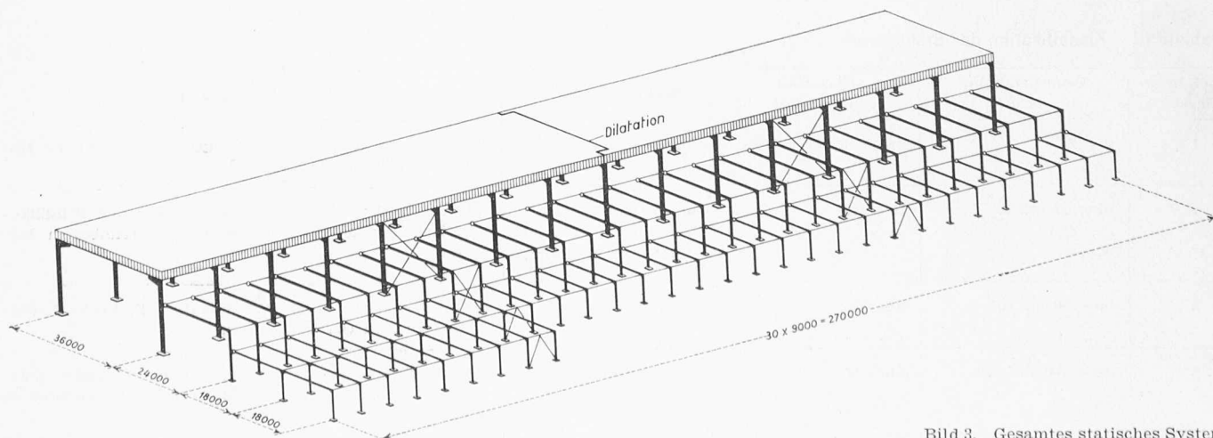
Bild 3. Gesamtes statisches System
